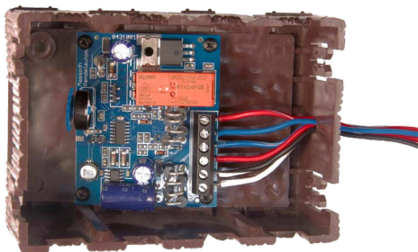
Abbildung 2: Einbau der Pendelautomatik in LGB Prellbock Nr. 10310
