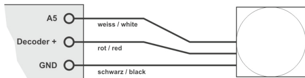
Abbildung 4: Anschluss eines Spannungspuffers
