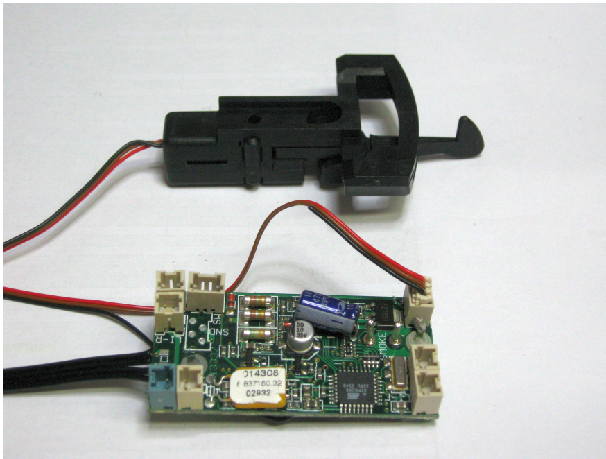
Abbildung 1: LGB OnBoard-Decoder klein von oben
