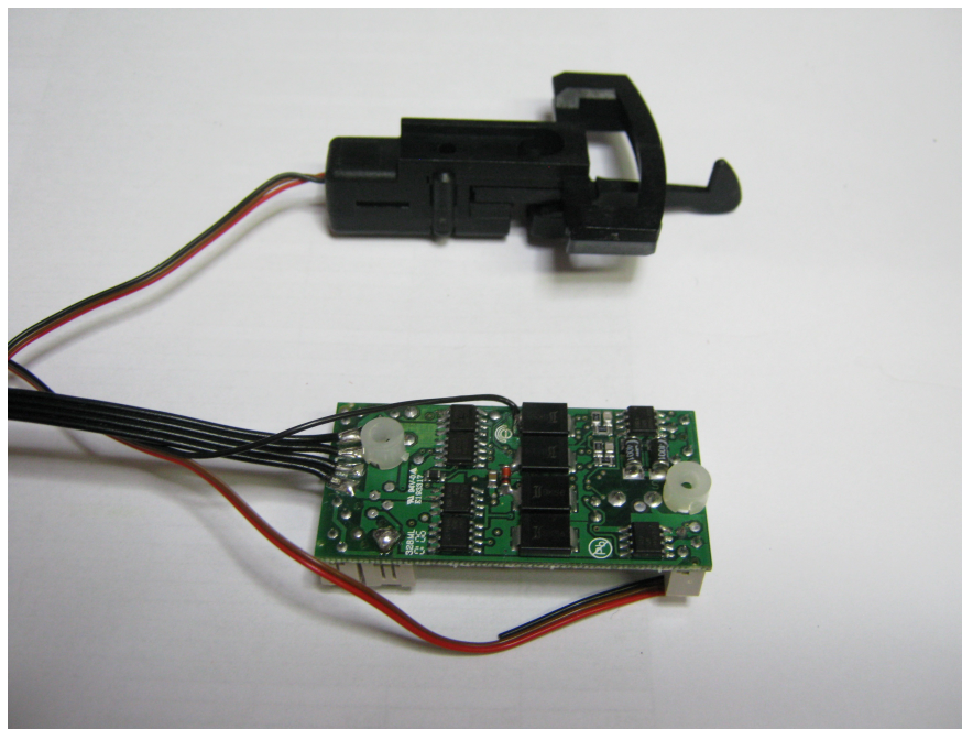
Abbildung 2: LGB OnBoard-Decoder klein von unten
