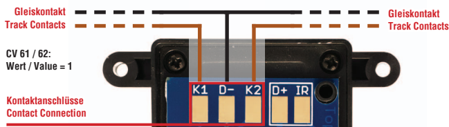
Abbildung 11: Verwendung der Kontaktanschlüsse als Eingang mit Gleiskontakten
