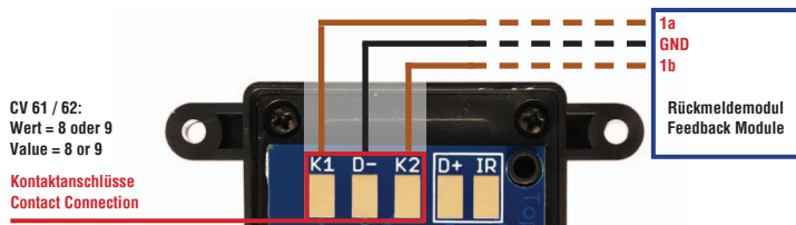
Abbildung 12: Anschluss des EVO-X an ein Rückmeldemodul (GND geschaltet)
