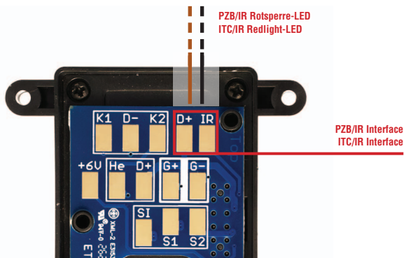
Abbildung 10: Anschluss PZB/IR Rotsperre LED als PZB/IR Signaldecoder
