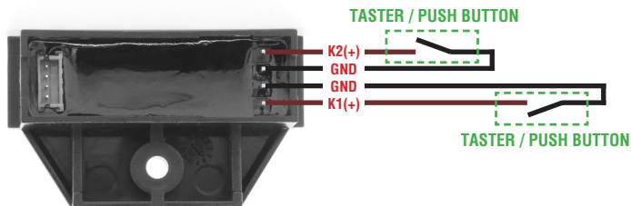
Abbildung 3: Schaltd decoder mit zwei angeschlossen Tastern
