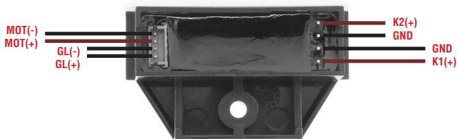
Abbildung 1: Schaltdecoder mit schematischer Anschlussdarstellung Figure 1: Switch Decoder with schematic connection scheme
