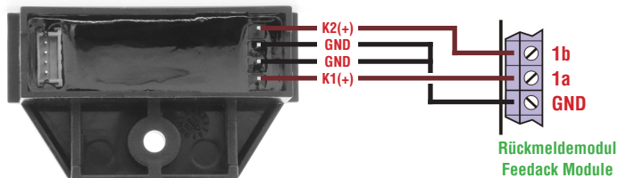
Abbildung 5: Schaltd decoder mit angeschlossenem Rückmeldemodul
