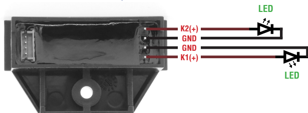
Abbildung 4: Schaltd decoder mit zwei angeschlossen LEDs
