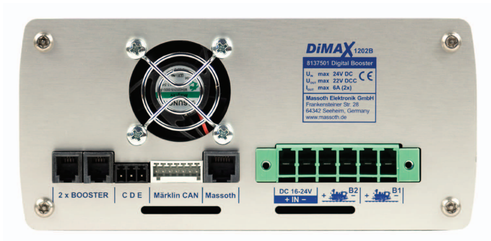
Abbildung 5: Anschlüsse auf der Rückseite des Booster 1202B Figure 5: Connections on the back side of the Booster 1202B
