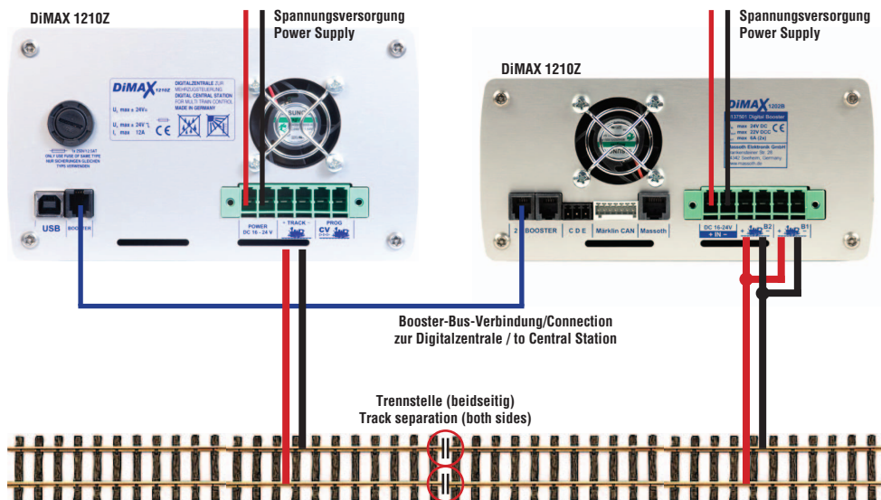
Abbildung 4: Anschluss der Trennstellen mit kombinierten Endstufen (je 12A) Figure 4: Arrangement of the separation points with joint power (12A each)
