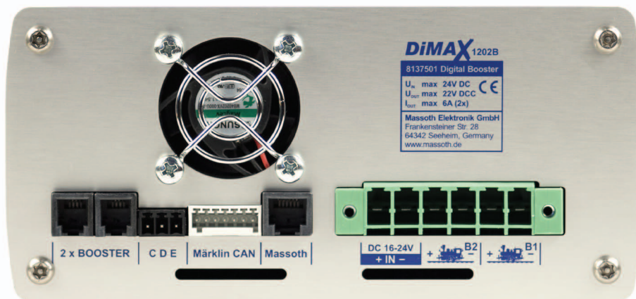
Abbildung 2: Anschlüsse auf der Rückseite des Booster 1202B Figure 2: Connections on the back side of the Booster 1202B
